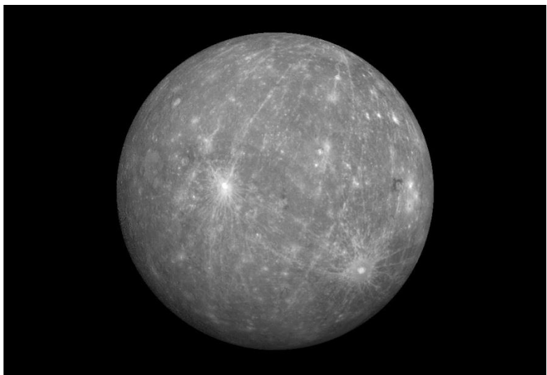
Mercurio
