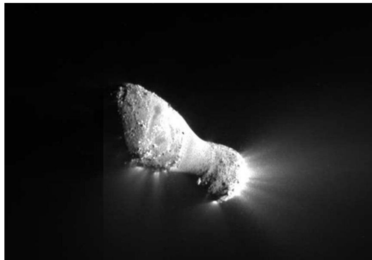
Nucleo cometario attivo
