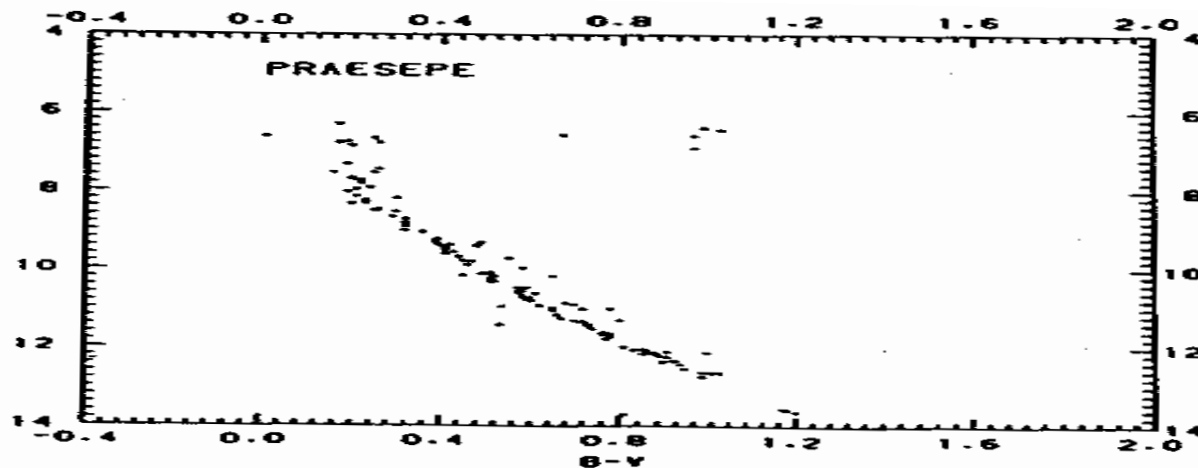
Diagramma HR
