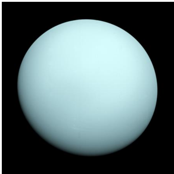
Urano
