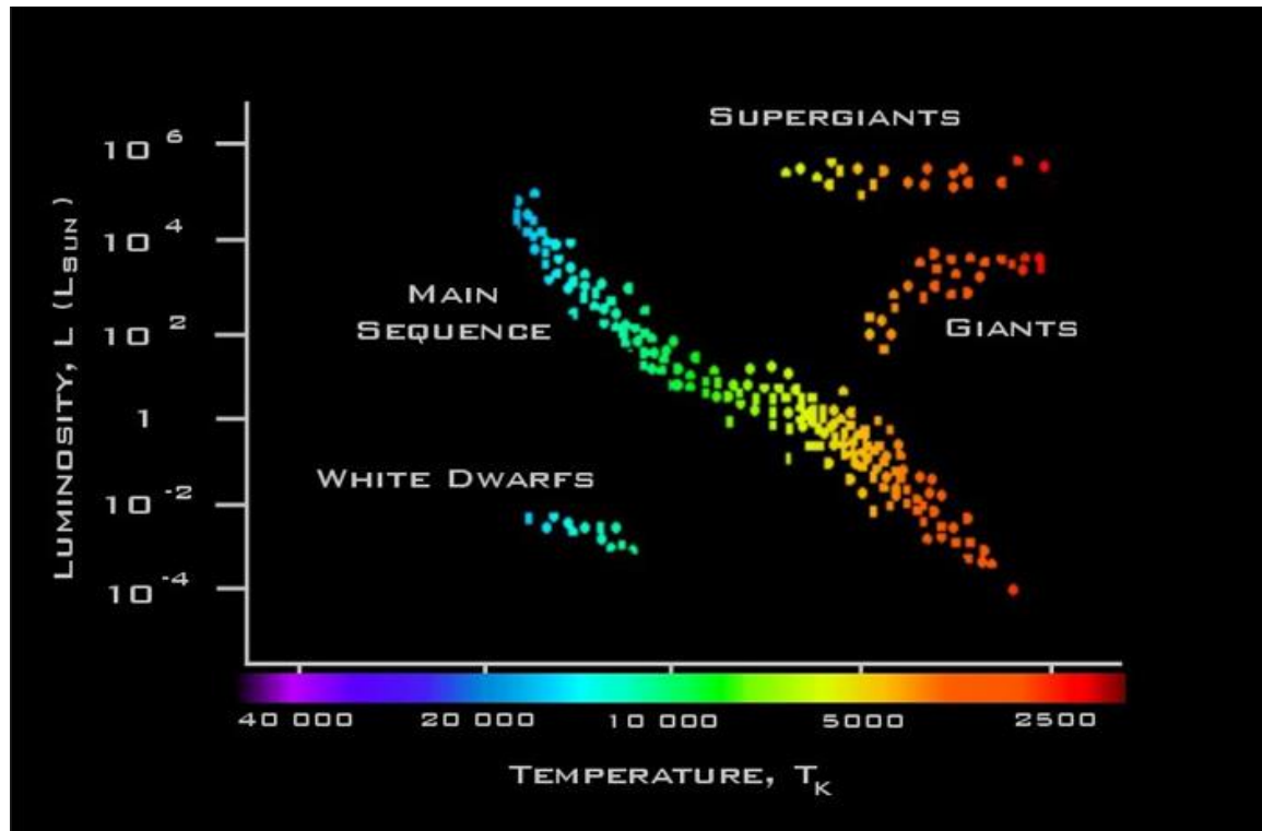
Diagramma HR
