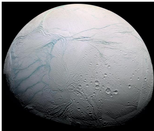
Encelado
