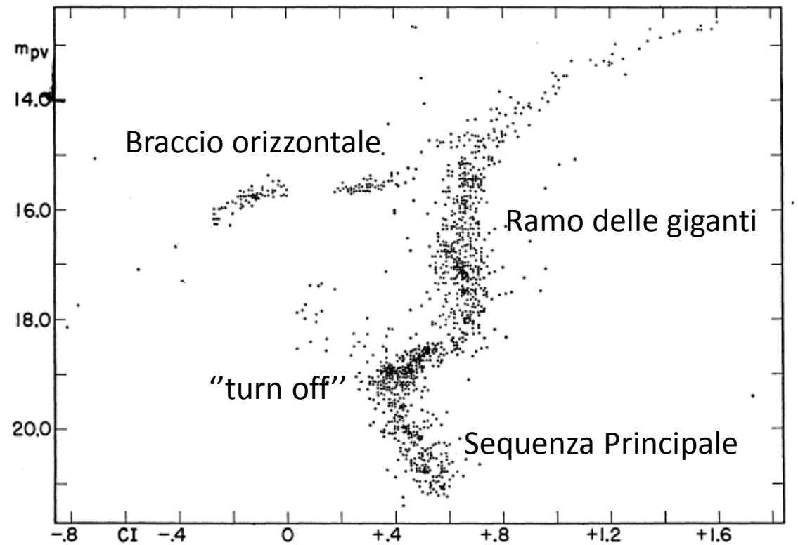
Diagramma HR ammasso globulare
