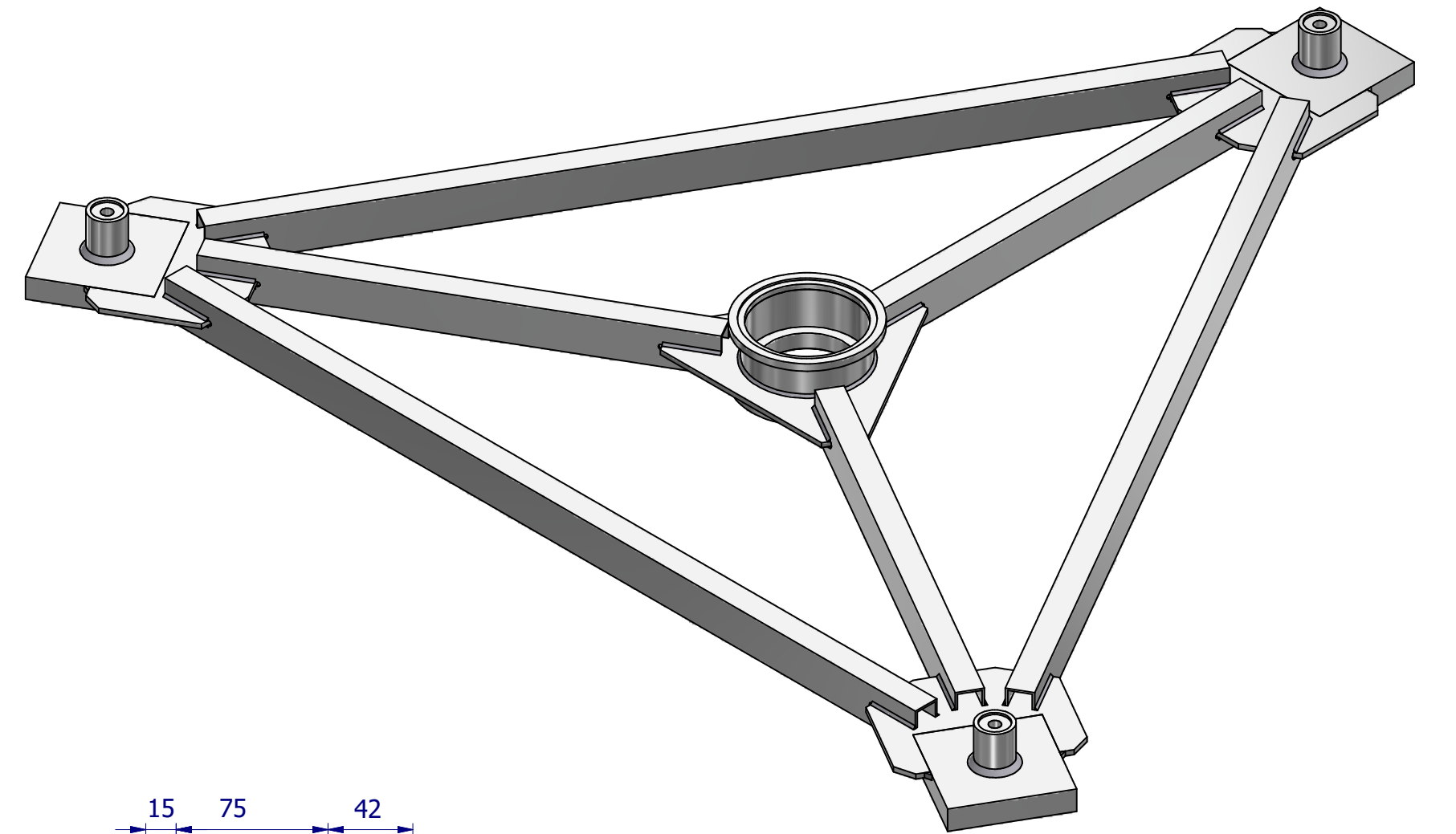
Dett. C
