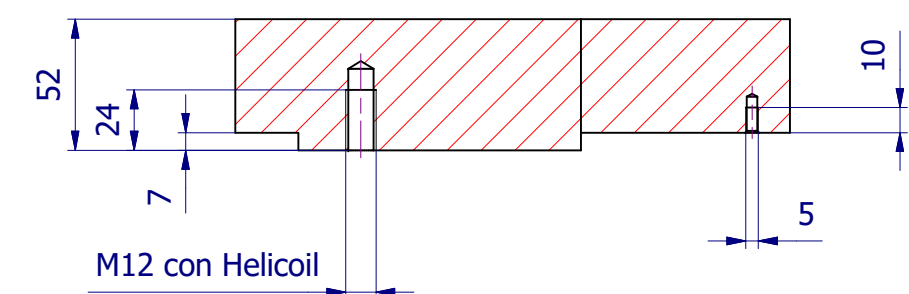
B-B
